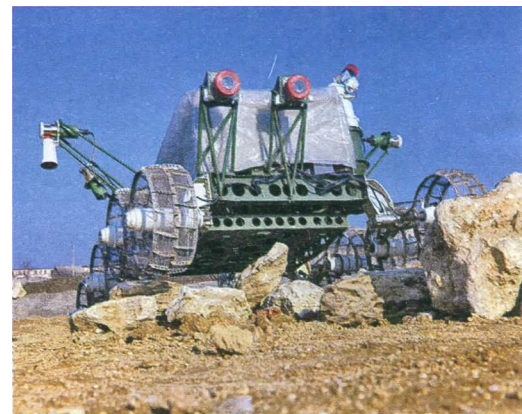
Испытание опытного образца первого лунного самоходного аппарата «Луноход-1»
